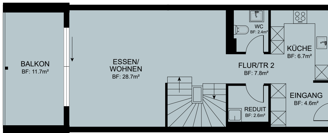
EBENE 2
